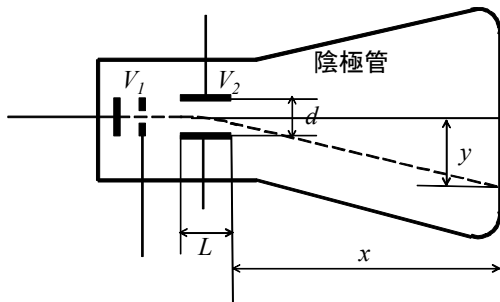
図1 偏向板入り陰極線管
